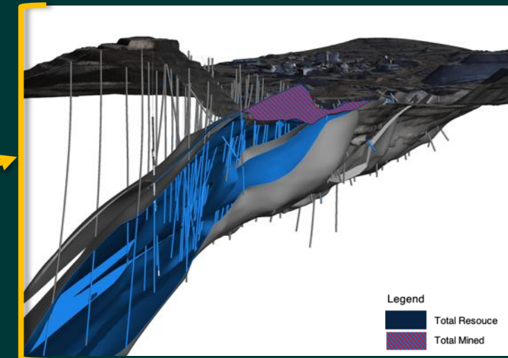
V1V2 Orebody
